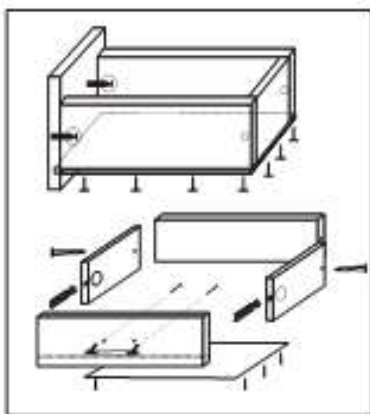
Сборка ящиков
